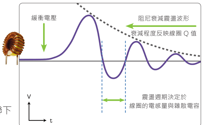
阻尼衰減波形進行比對分析
