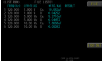
多步列表：施加不同 DC Bias 電壓量測出電容值變化
