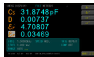
Meter 模式下監測 \epsilon_r' / \epsilon_r''
